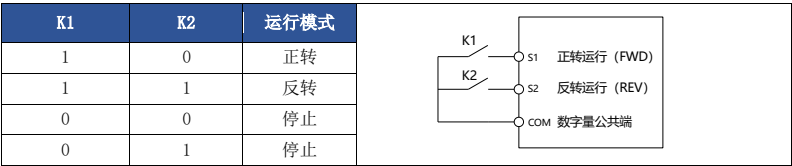
图 6-9 两线式模式 2
