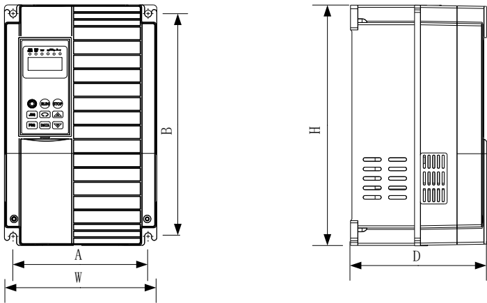
图 2-3 变频器壁挂安装示意图
