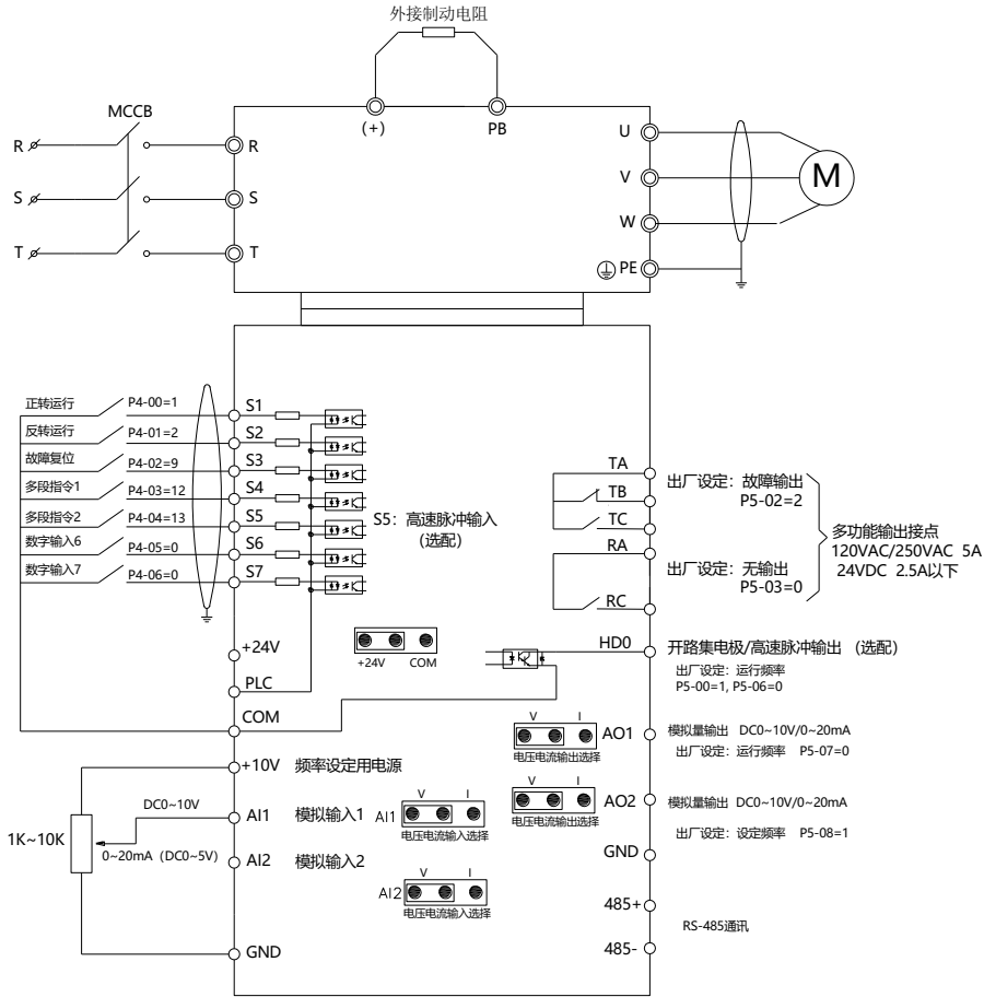
图 3-4 标准接线图
