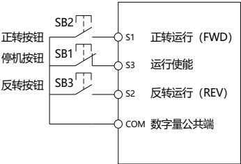
图 6-10 三线式控制模式 1
